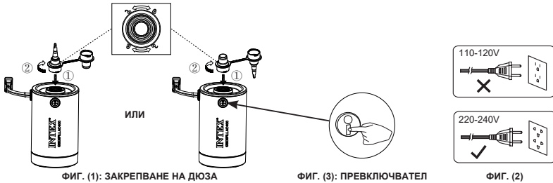
ФИГ. (1): ЗАКРЕПВАНЕ НА ДЮЗА
